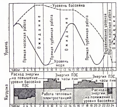
Рис. 1. График внутрисуточного регулирования режима работы ПЭС (пример).
